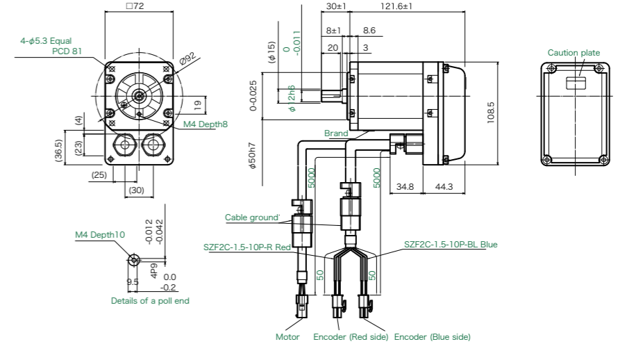
● 200W タイプ AC サーボモータ
