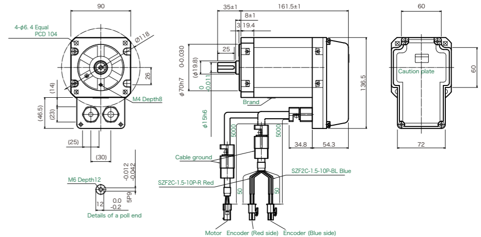
● 600W タイプ AC サーボモータ
